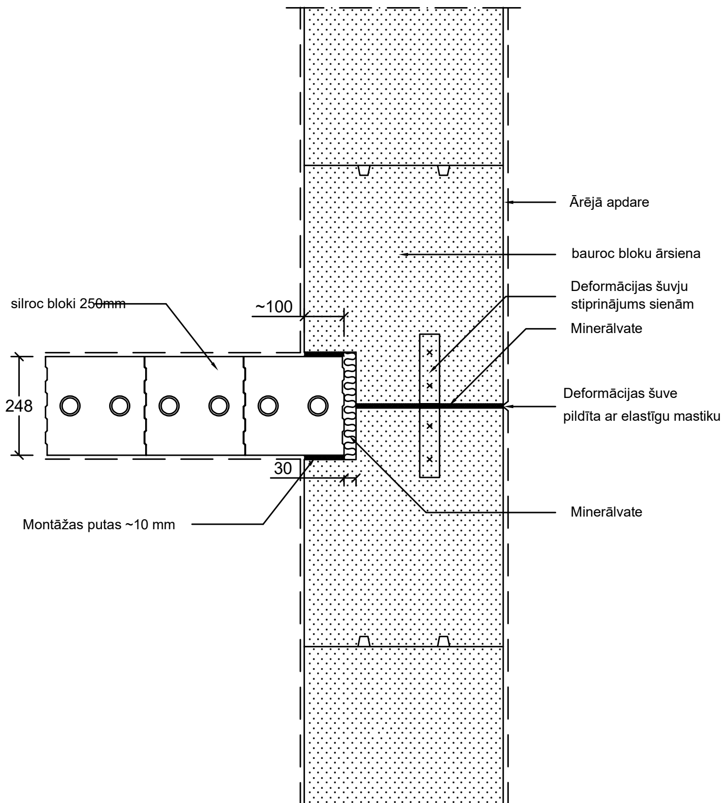
Silroc sienas skaņas izolācija R'w \geq 55\text{dB} (ar apdari)
